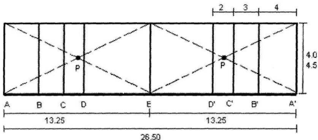
Рис. 2. Разметка площадки.
